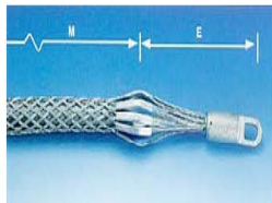
旋转头拉线网套连接器 旋转头拉线网套连接器
